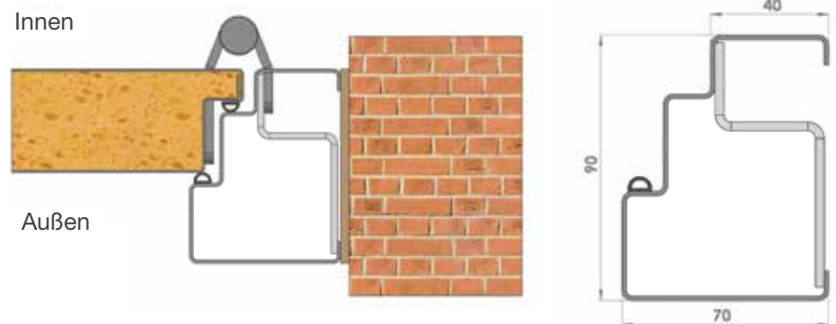
GEHRUNGSRAHMEN, ÖFFNUNG NACH INNEN ( LI )
