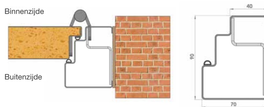
VERSTEKFRAME MET AANSLAG, BINNENDRAAIEND (LI)
