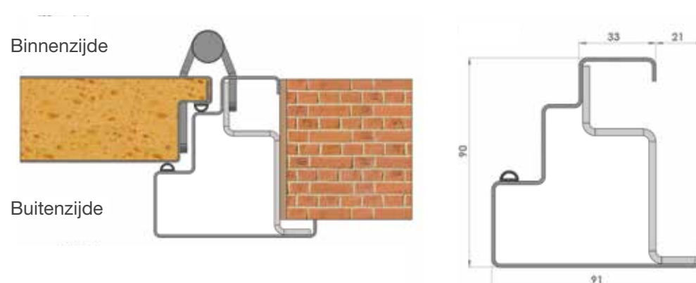
VERSTEKFRAME MET AANSLAG, BINNENDRAAIEND (MI)
