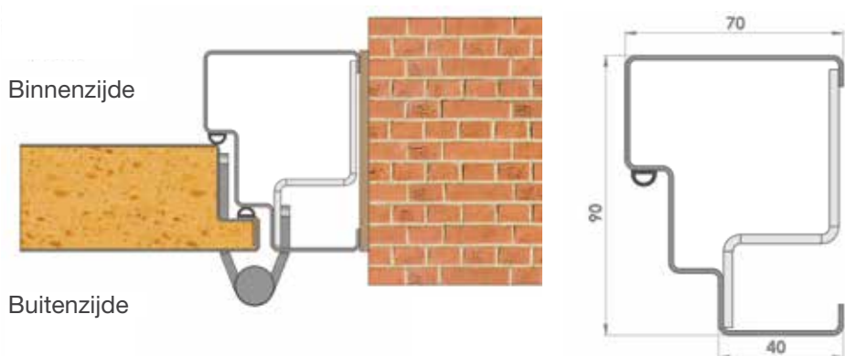
VERSTEKFRAME MET AANSLAG, BUITENDRAAIEND (LO)
